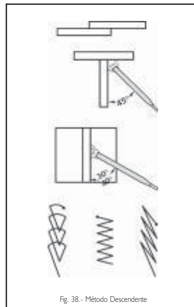
Fig. 38.- Método Descendente
