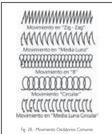
Fig. 28.- Movimiento Oscilatorios Comunes
