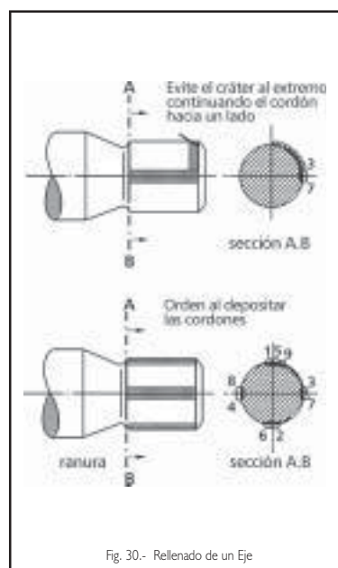
Fig. 30.- Rellenado de un Eje
