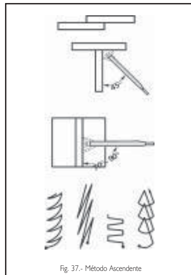
Fig. 37.- Método Ascendente
