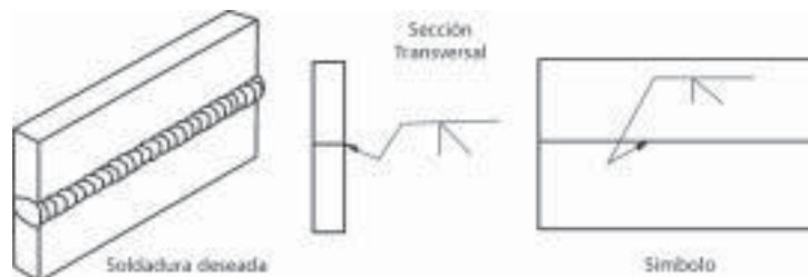
Fig. 75.- Símbolo de la Soldadura a Tope con Chafán en el Lado Próximo a la Flecha
