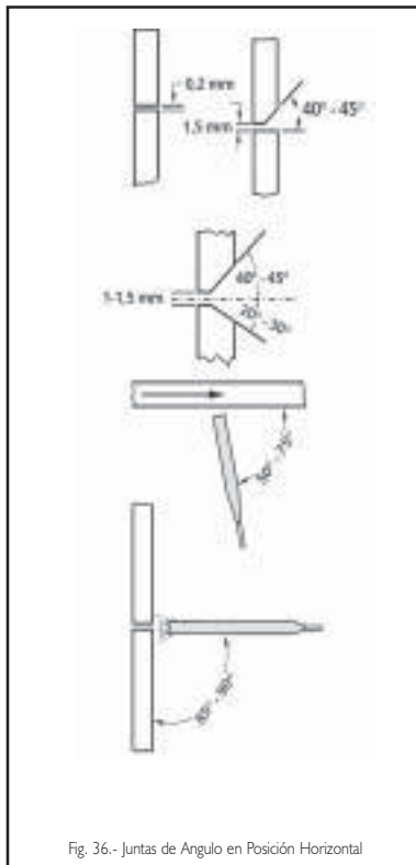
Fig. 36.- Juntas de Angulo en Posición Horizontal
